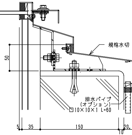
角型タイプ断面
